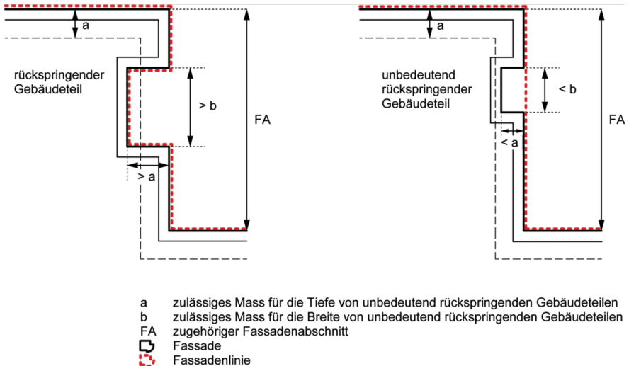
Figur 3.5 Rückspringende und unbedeutend rückspringende Gebäudeteile
