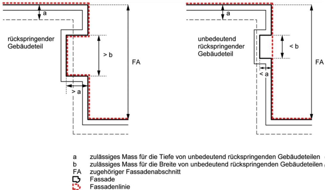
Figur 3.5 Rückspringende und unbedeutende rückspringende Gebäudeteile
