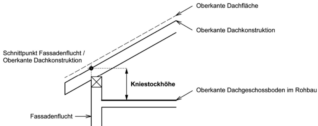
Figur 5.3 Kniestockhöhe
