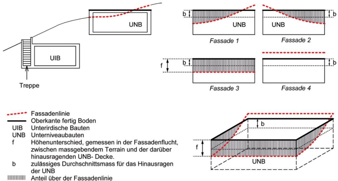
Figur 2.4 und 2.5 Unterirdische Bauten, Unterniveaubauten
